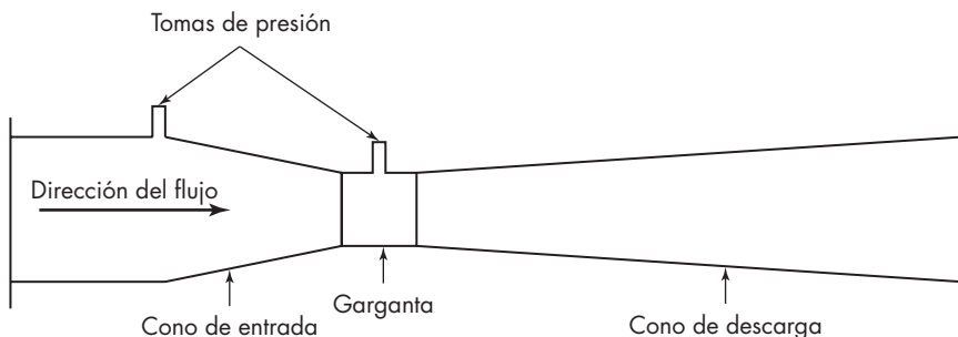
FIGURA 8.16 Medidor venturi.
